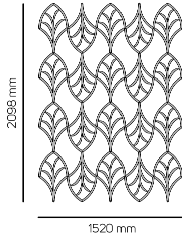
Opstelling 2 Leaf 2D Bestaande uit 20 onderdelen
