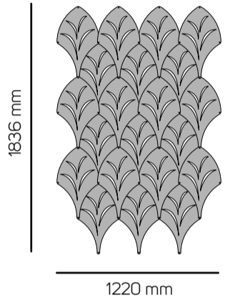
Opstelling 1 Leaf 3D Bestaande uit 21 onderdelen
