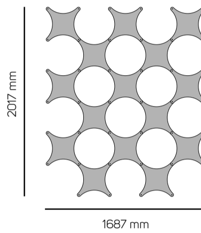
Opstelling 3 Cross Bestaande uit 15 onderdelen
